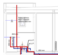
CORTE B-B'
