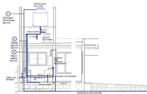
CORTE C-C'
