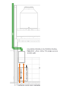
CALDERA TIPOLOGIA V1A
