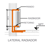
LATERAL RADIADOR
