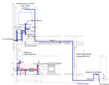
CORTE A-A'
